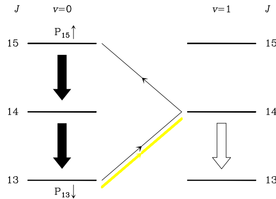
FIGURA 5.5. – Mecanismo de bombeo para los máseres M_2 y M_3 . El solapamiento entre las líneas SiS R(13) y C_2H_2 \nu_5(\pi_u) - G.S.(\sigma_g^+) R_e(9) aumenta significativamente la población en el nivel v = 0 J = 15 reduciendo a su vez la población del nivel v = 0 J = 13 . De este modo es posible la aparición de los máseres M_2 y M_3 . Durante el proceso también aumenta la población del nivel v = 1 J = 14 , que podría generar un máser no observado en la transición v = 1 J = 14 - 13 .
