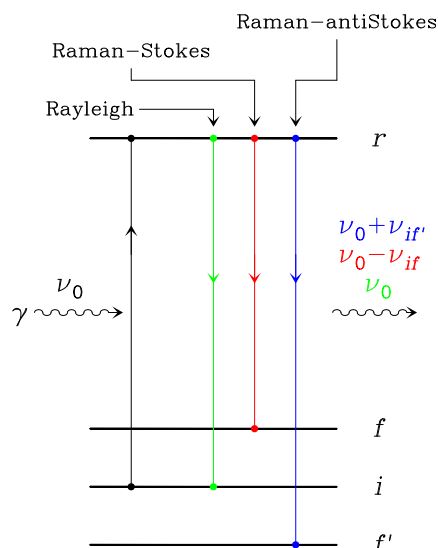
FIGURA 10.1. — Esquema de la dispersión Raman cuántica. Un fotón excita una molécula del nivel i al metaestable r que se desexcita espontáneamente. Esa desexcitación puede llevar a la molécula de nuevo al nivel i (dispersión Rayleigh; verde), al nivel f (dispersión Raman-Stokes; rojo), o al nivel f' (dispersión Raman-antiStokes; azul).
