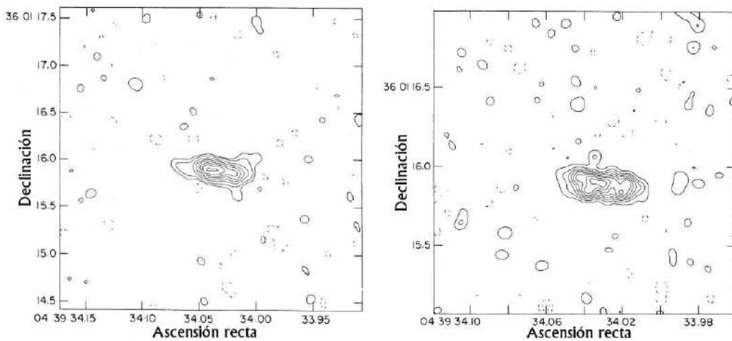
FIGURA 1.17.— Observaciones interferométricas de CRL618 realizadas con el VLA. Ambos mapas corresponden al continuo emitido por la región HII. El de la izquierda está tomado a 2 cm con un haz de 0^{\circ}.12 mientras que el mapa de la derecha muestra el continuo a 1.3 cm observado con un haz de 0^{\circ}.07 (Figura tomada de Kwok & Bignell, 1984).
