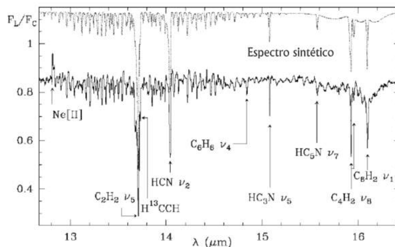
FIGURA 1.20.— Espectro infrarrojo de CRL618 tomado con SWS/ISO. Se observan claramente bandas en absorción de varias especies moleculares como son los poliinos C_4H_2 y C_6H_2 , los cianopoliinos HC_3N y HC_5N y el benceno ( C_6H_6 ). En la figura se incluye un ajuste al espectro observado obtenido mediante la aplicación del código LVG desarrollado por J. Cernicharo (Figura tomada de Cernicharo et al., 2001a ).
