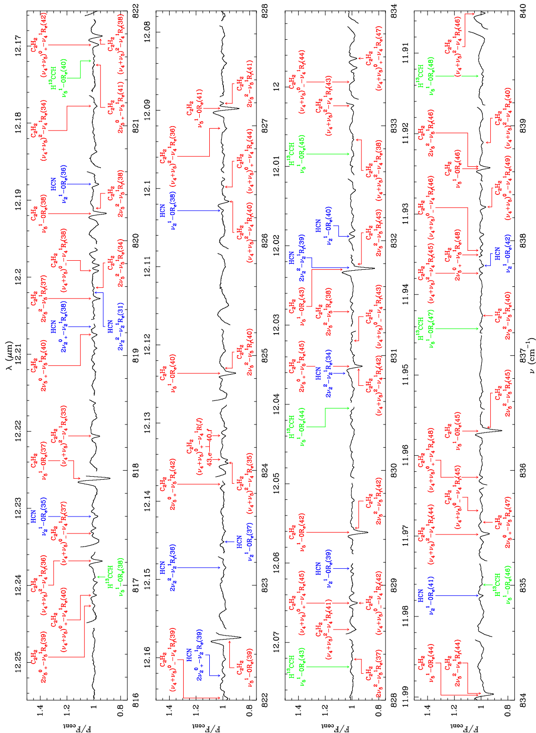
FIGURA 4.5. — Espectro observado de IRC+10216 en el intervalo 816\text{--}840\text{ cm}^{-1} con resolución de \approx 10^{-2}\text{ cm}^{-1} ( \approx 3\text{--}4\text{ km s}^{-1} ). En la Figura se indican las transiciones más importantes de \text{C}_2\text{H}_2 (rojo), HCN (azul), \text{H}^{13}\text{CCH} (verde) y \text{H}^{13}\text{CN} (azul claro). La escala del eje y ha sido cambiada con respecto a las Figuras 4.1-4.3 para mostrar las líneas moleculares más claramente.
