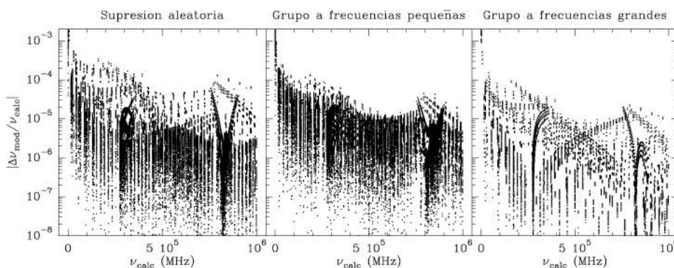
FIGURA C.8. — Estudio de estabilidad de las frecuencias calculadas ( \text{CH}_2\text{CN} ). Para conocer el significado de las gráficas y los estudios que representa cada una, léase la nota de la Figura C.2 y el texto. Las frecuencias calculadas parecen lo suficientemente estables como para no sufrir grandes modificaciones al añadir más frecuencias experimentales al conjunto inicial. La supresión aleatoria es el proceso que parece generar más inestabilidad mientras que los otros dos dan lugar a comportamientos similares, siendo únicamente las frecuencias por debajo de 30 GHz las susceptibles de pasar de la zona de buena calidad a las zonas de calidad aceptable o deficiente. Por encima de 40 GHz, todas las frecuencias modificadas están en la zona de buena calidad o calidad aceptable.
